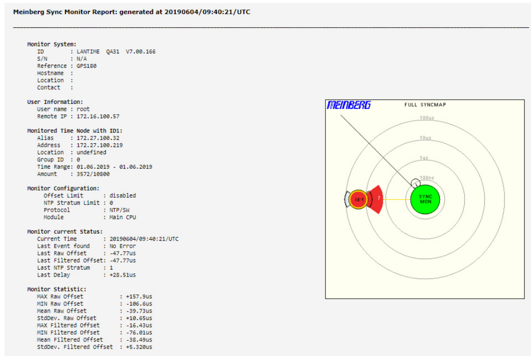
Abbildung: Generierter Bericht für ausgewählte Knoten in der Tabelle. Der Bericht enthält Statusinformationen über die ausgewählten überwachten Knoten, die Monitorkonfiguration, die Hauptmonitorstatistiken und grafische Diagramme.
