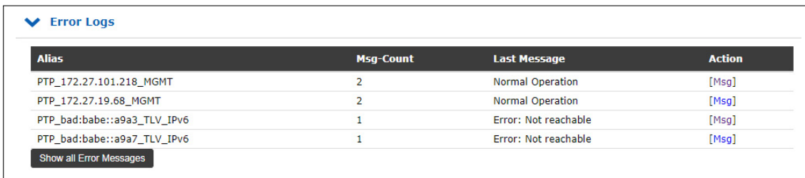
Abbildung: Fehlerprotokoll-Statistik.
