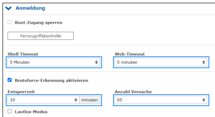
Abbildung 7.10: Timeout der Webschnittstelle einstellen
